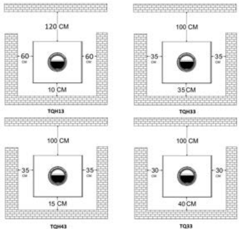
Abb. 1. Sicherheitsabstände
