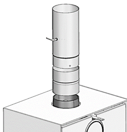
Fig. 12.- Exemple d'installation d'un régulateur du tirage
